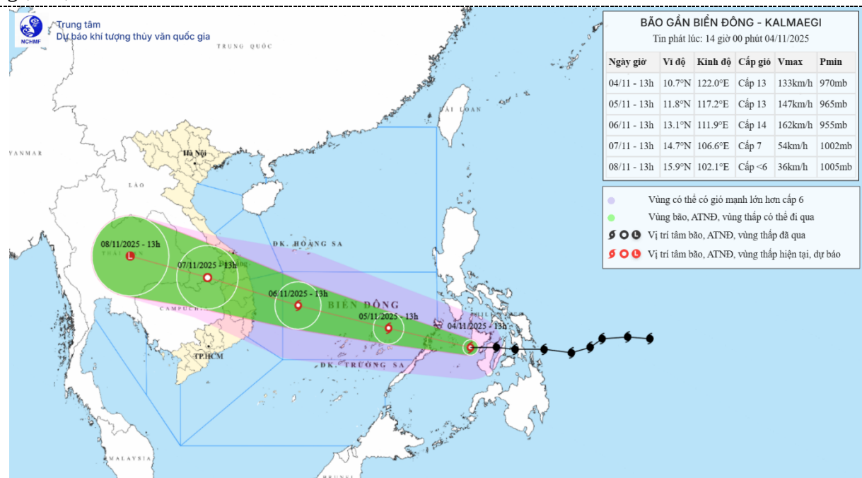
Hình 1. Bản đồ dự báo quỹ đạo và cường độ bão KALMAEGI phát lúc 14h00 ngày 04/11/2025.
